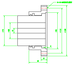
冷剪后辊道电机端鼓型齿联轴器
