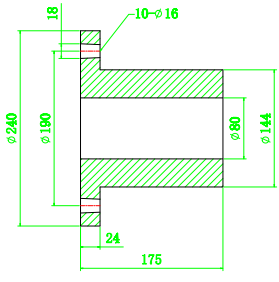
空烟风机联轴器
